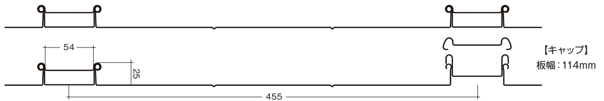
【丸ハゼ式瓦棒】
